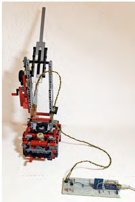
Magnetfeldsucher von Lars und Oleksandra, JuFo25.
