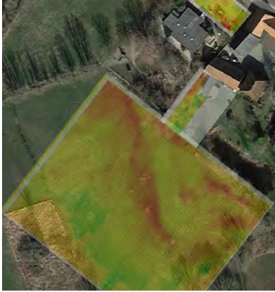
Geophysikalische Messung auf einer Wiese bei Thune – Unter der Erde befinden sich, noch unsichtbar, die Überreste einer mittelalterlichen Burg (rötliche Bereiche).
